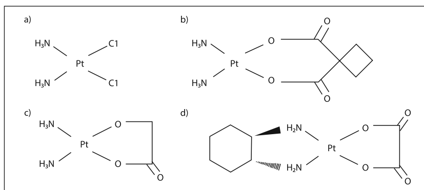
Rycina 1. Wzory strukturalne leków platynowych: a) cisplatina, b) karboplatyna, c) nedaplatyna, d) oksaliplatyna
