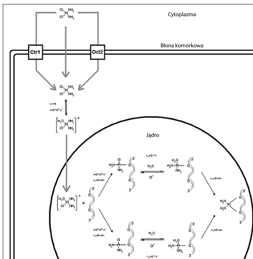
Rycina 3. Aktywacja, kinetyka i transport cisplatyny z przestrzeni międzykomórkowej do wnętrza komórki
