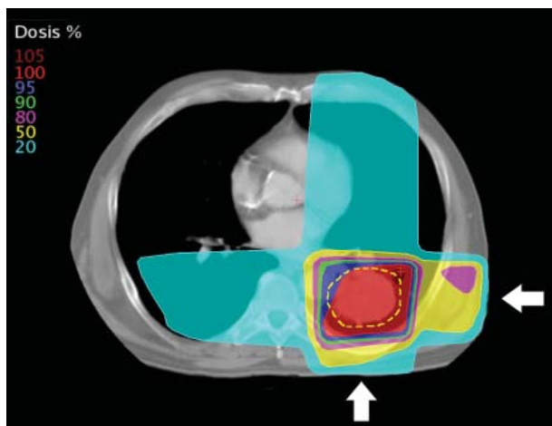
Ryc. 7. Fotonowy
