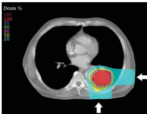
Ryc. 8. Protonowy
