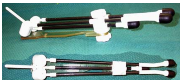
Ryc. 3. Kompatybilne z MRI/CT tandem i aplikatory pochwowe z ovoidami
