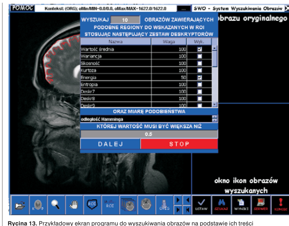
Rycina 13. Przykładowy ekran programu do wyszukiwania obrazów na podstawie ich treści
