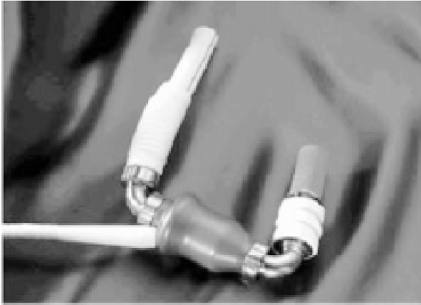
Rycina 4. HeartMate II — pompa wspomagająca pracę lewej komory
