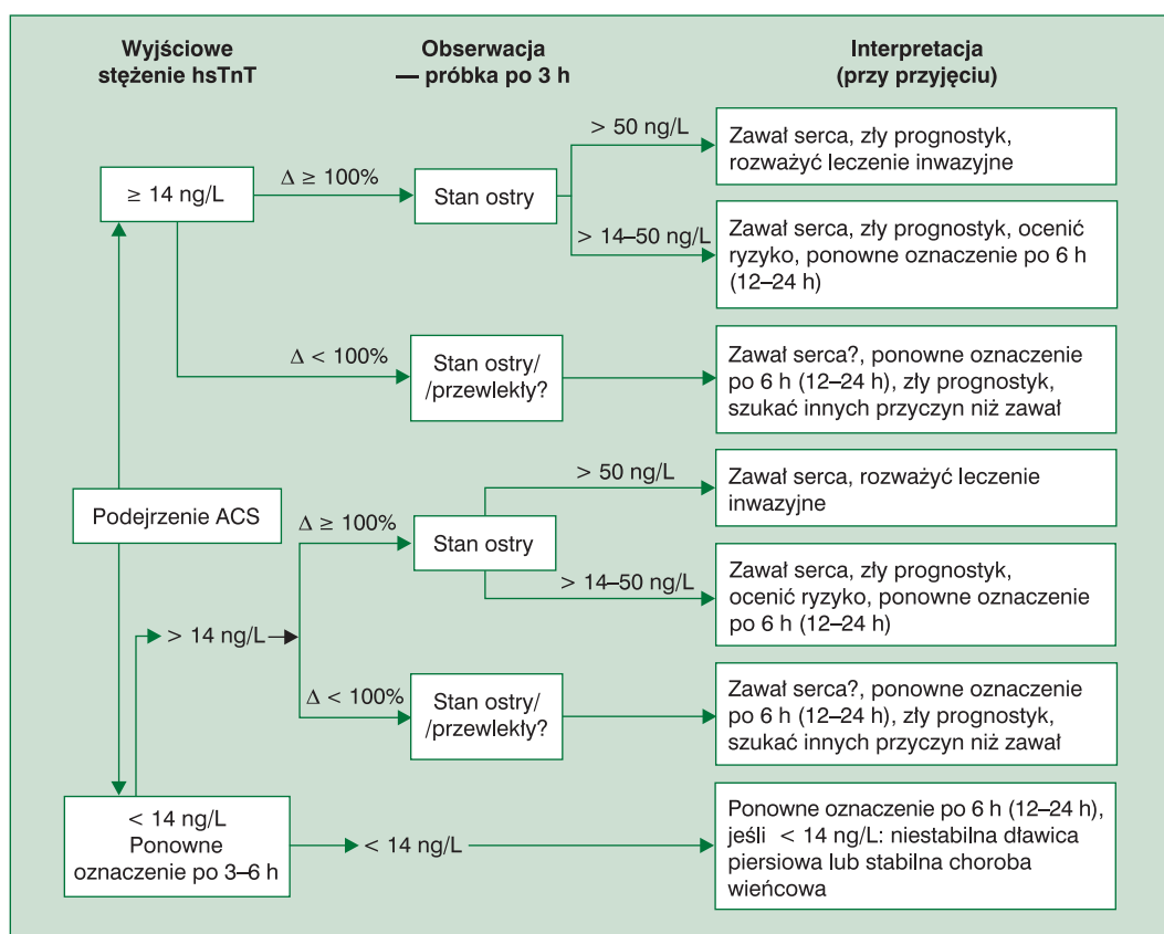
Rycina 1. Algorytm interpretacji stężenia wysoce czulej troponiny T (hsTnT, high-sensitivity troponin ) w praktyce klinicznej; ACS ( acute coronary syndrome ) — ostry zespół wieńcowy
