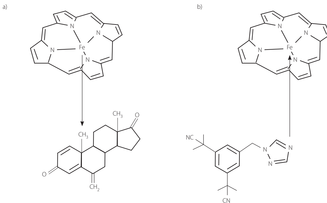
Rycina 4. Odziaływanie steroidowych i niesteroidowych inhibitorów z centrum aktywnym aromatazy – a) eksmestan, b) anastrozol
